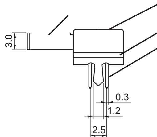
1A DETAIL
